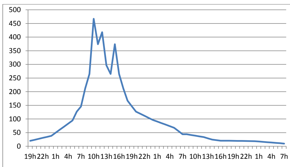
Figure 19: Hydrogramme de la crue du 11/02/1987 en m 3 /s
