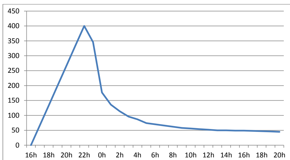
Figure 20: Hydrogramme de la crue du 17/08/1995 en m3/s
