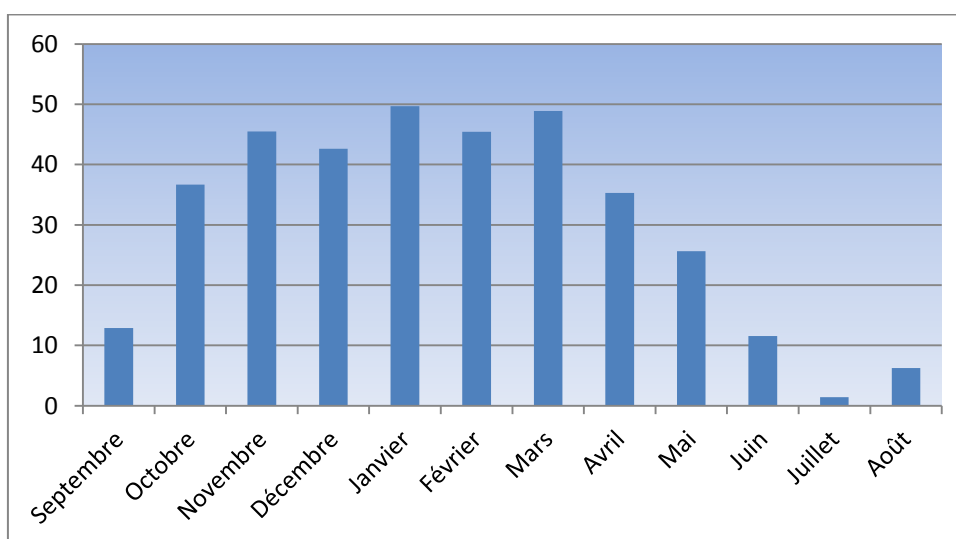
Figure 9: Histogramme de précipitations moyennes mensuelles au niveau de bassin versant Zat
